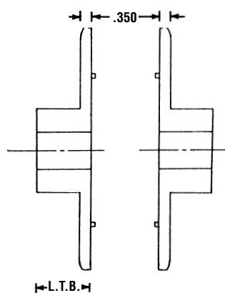
Tipo B (Hierro Fundido)
