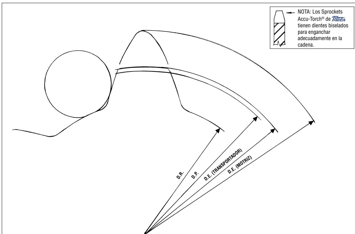
Diente Tipo Transportador para Cadenas: 78 — 82 — 124 — 132
